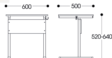
Парта регулируемая, односторонняя Ш-301(4-6)
