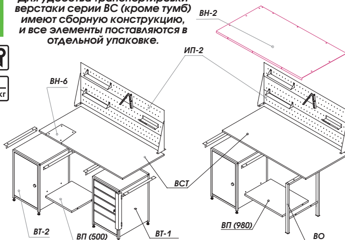
Верстак в базовой комплектации ВС-3
