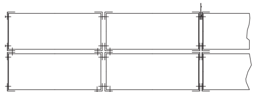
Рекомендуемая схема сборки Ст-12
