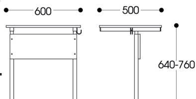
Парта регулируемая с механизмом подъема столешницы Ш-301М (4-6)
